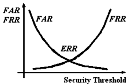
Fig. 13: FAR-FRR Rate [24].
